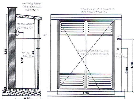
CORTE CASILLA DE GAS ES: 1:20
