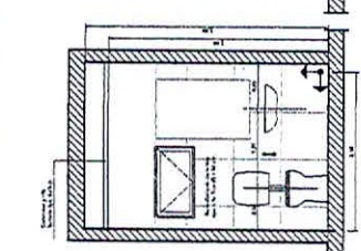
VISTA BAÑO B-B
